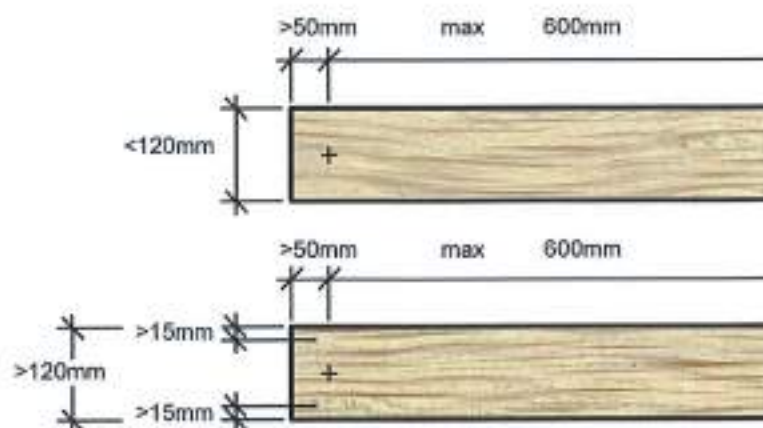
Tekening 9 Moatvoering bevestigingspunten.
