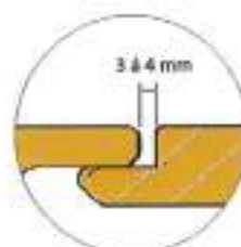
Tekening 10 Vol- doende expansie- ruimte aanhouden tussen delen.
