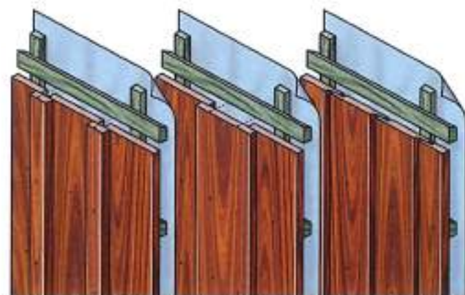
Tekening 3 Verticale gevelbekleding: v.l.n.r. opdekwerk, opdekwerk en rabat met halfhoutse overlap (Chanel siding).
